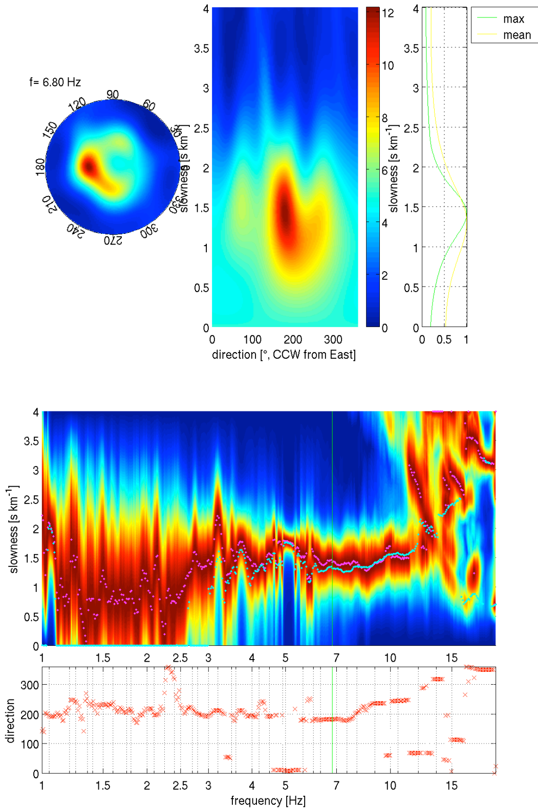
Abbildung B.1. : F-K Analyse und Dispersionskurve für Ring mit 20-50 m Radius.
