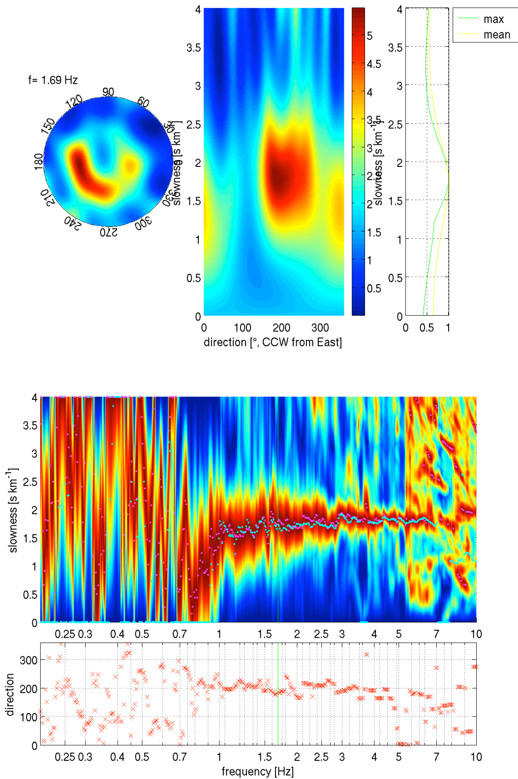
Abbildung B.2. : F-K Analyse und Dispersionskurve für Ring mit 100-200 m Radius.
