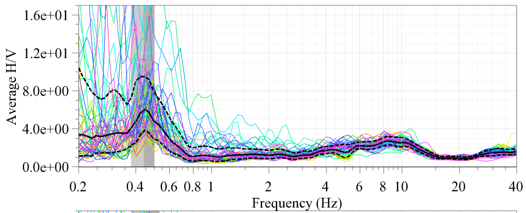
Abbildung 4. Resultat der H/V Polarisationsanalyse der Stationen im Array Sioo.
